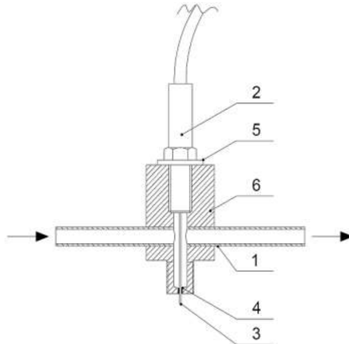
Rys. 4. Przekrój poprzeczny termopary typu K umieszczonej w płaszczu wodnym:
