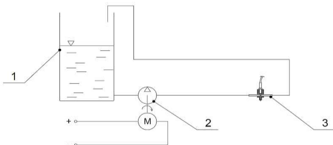
Rys. 5 Schemat ideowy układu chłodzenia termopary:
