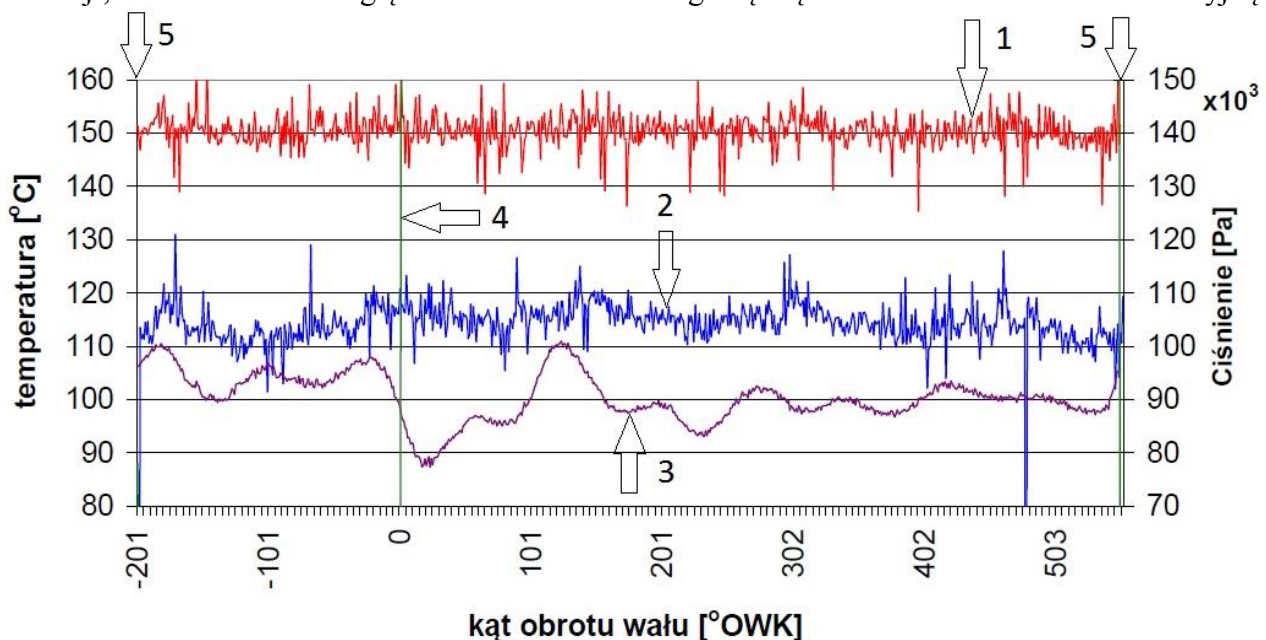
Rys. 3. Przebiegi zmienności temperatur zarejestrowanych w kanale wylotu spalin silnika Farymann Diesel typu D10 rejestrowane dwoma termoparami typu K podczas jednego cyklu pracy; 1 - temperatura rejestrowana termoparą odkrytą, 2 - temperatura rejestrowana termoparą chłodzoną wodą, 3 - ciśnienie w kanale spalin wylotowych, 4 - sygnał zamknięcia zaworu wylotowego, 5 - sygnał otwarcia zaworu wylotowego
