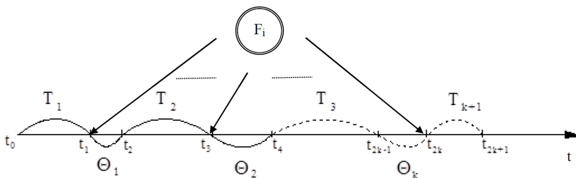
Rys. 3 Proces eksploatacji, jako sekwencja zdarzeń - przykład. Przedział [t_0, t_1] - czas zdatności silnika do pierwszego uszkodzenia (zmienna losowa T_1 ), przedziały (t_2, t_3), \dots, (t_{2k}, t_{2k+1}) - czasy zdatności silnika pomiędzy kolejnymi uszkodzeniami (zmiennne losowe T_2, T_3, \dots, T_{k+1} ), przedziały (t_1, t_2), \dots, (t_{2k-1}, t_{2k}) - czasy odnowienia stanu zdatności silnika (zmiennne losowe \Theta_1, \Theta_2, \dots, \Theta_k ), suma długości przedziałów (t_2, t_3), \dots, (t_{2k}, t_{2k+1}) - sumaryczny czas stanu zdatności silnika (zmienna losowa T ), suma długości przedziałów (t_1, t_2), \dots, (t_{2k-1}, t_{2k}) - sumaryczny czas trwania stanu niezdatności (czasu odnowienia) silnika (zmienna losowa \Theta )
