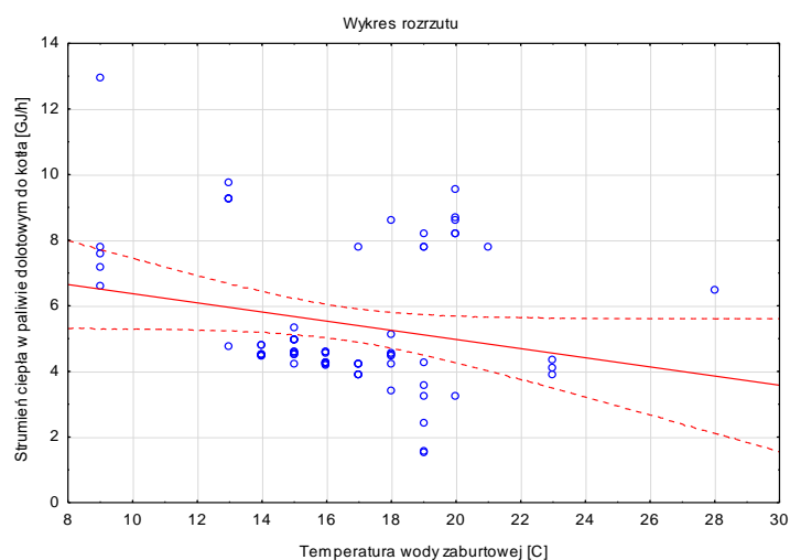
Rys. 2 Wykres korelacji strumienia ciepła do kotła a temperaturą wody zaburtowej
